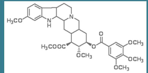
Fórmula química de la Reserpina
